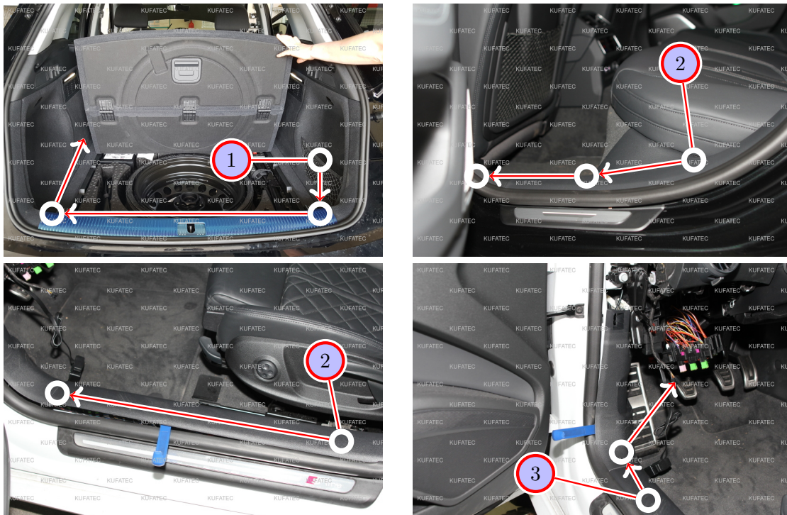
Abbildung 5: Verlegung Tasterkabel
