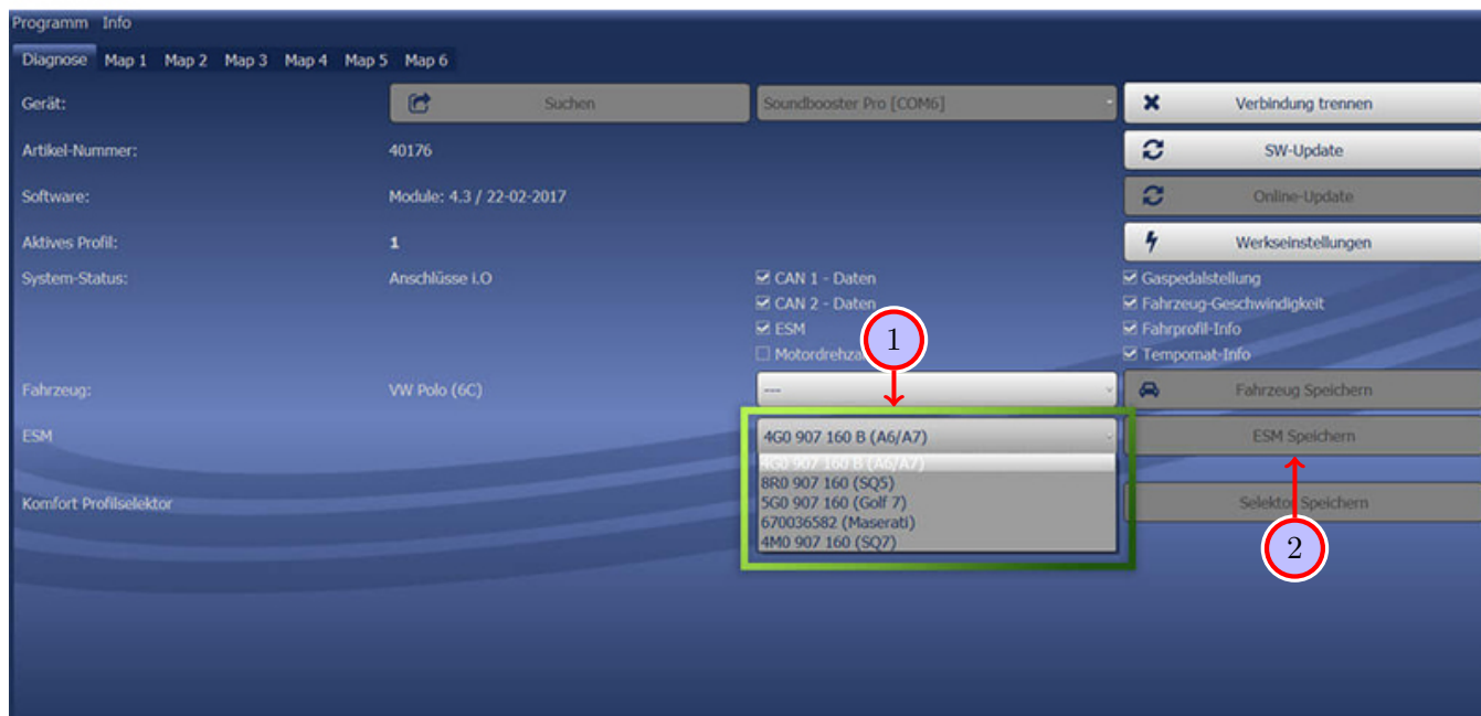
Abbildung 8: Software
