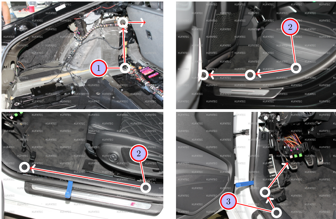
Abbildung 6: Verlegung Tasterkabel
