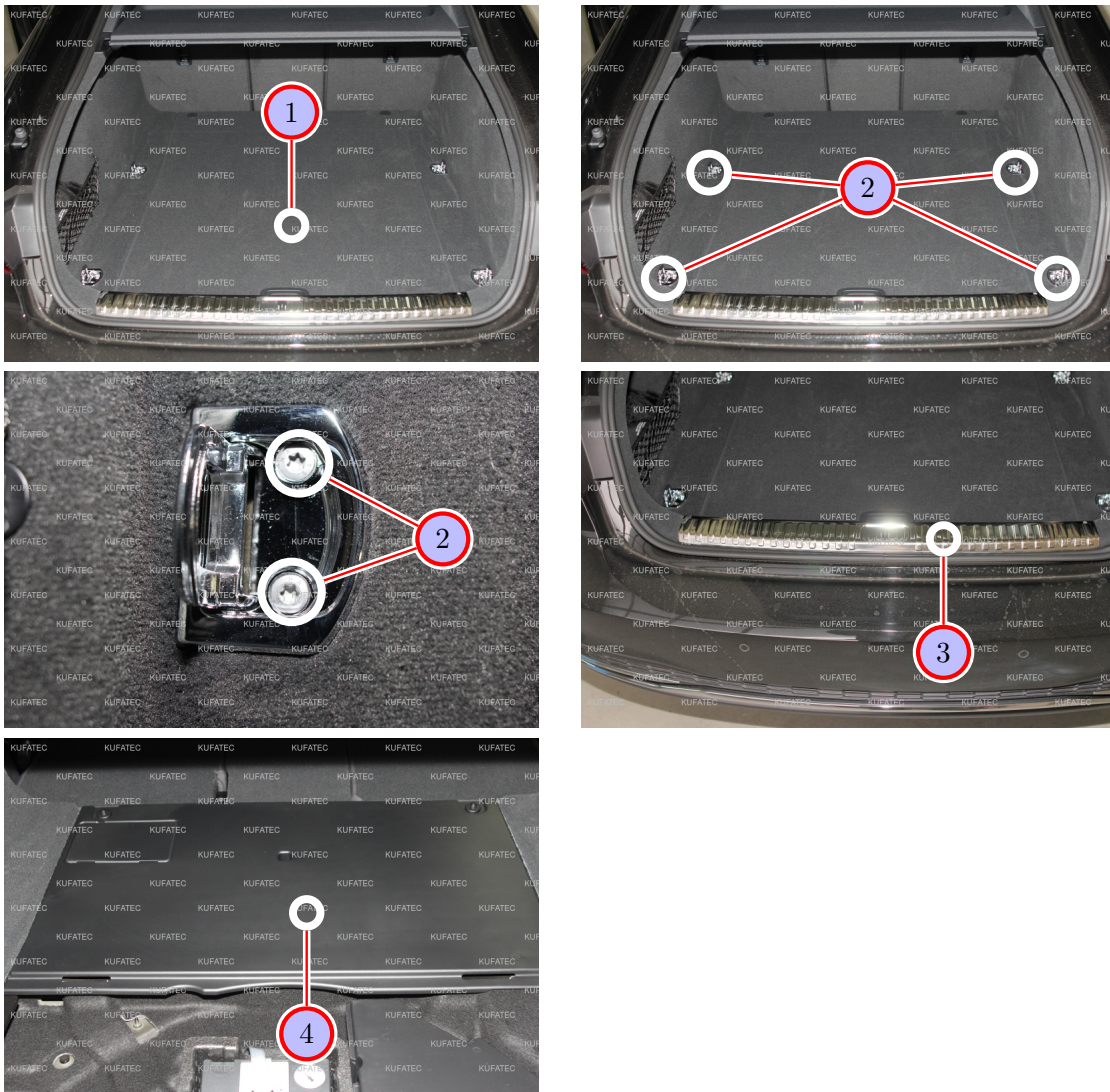
Abbildung 4: Demontage Kofferraum
