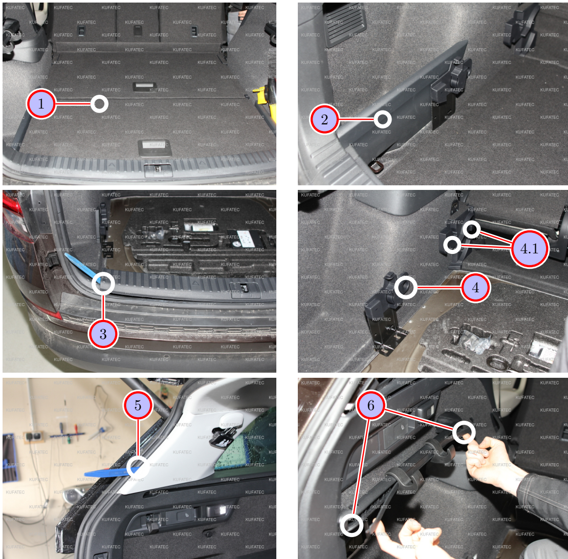
Abbildung 4: Demontage Verkleidung Kofferraum
