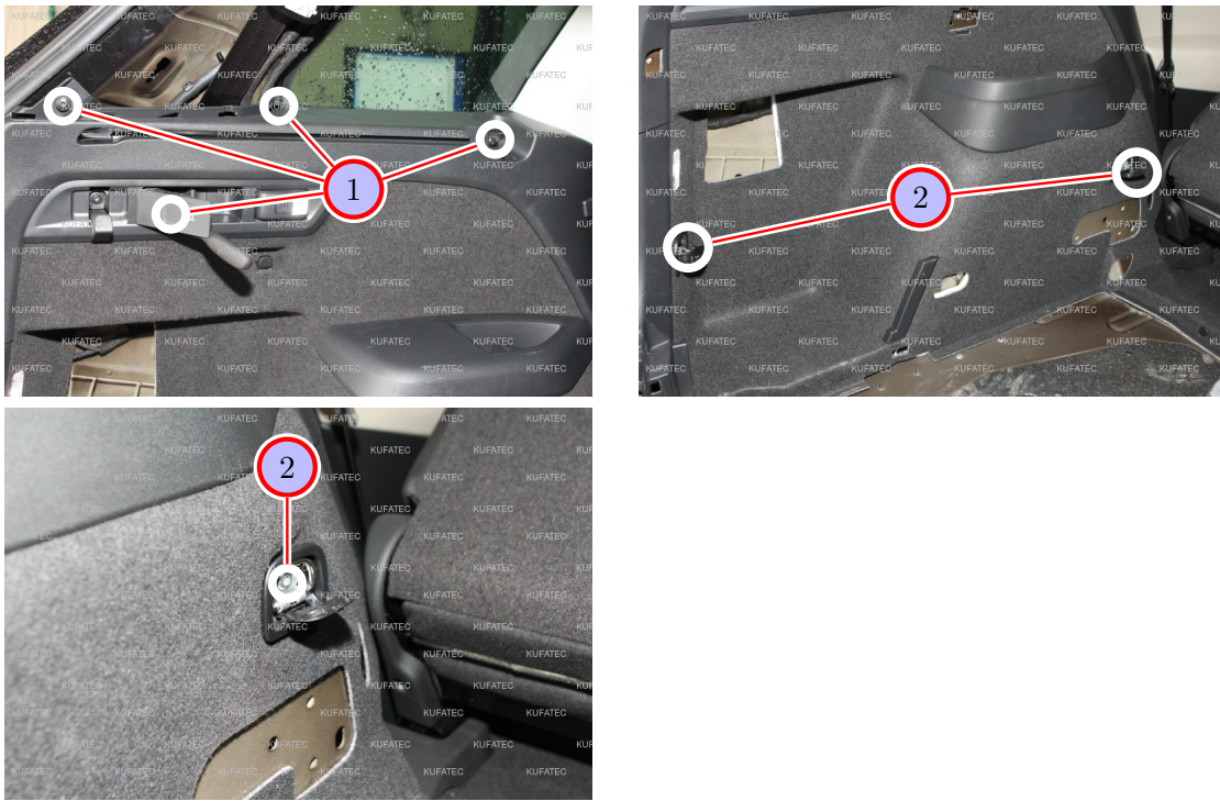
Abbildung 5: Demontage Verkleidung Kofferraum
